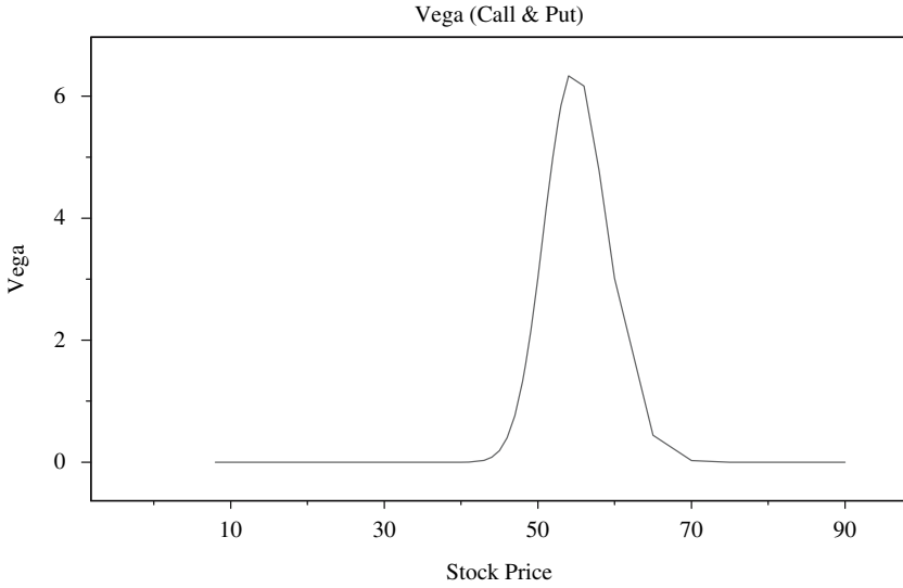
FIGURE 10.11. Vega.
